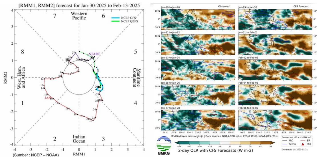
Gambar 10. Pergerakan MJO 23 Januari 2025 – 3 Maret 2025 (kiri) dan Total Rata-rata dan Anomali OLR 01 Februari 2025 – 03 Maret 2025 (kanan) (sumber: www.bom.gov.au )
