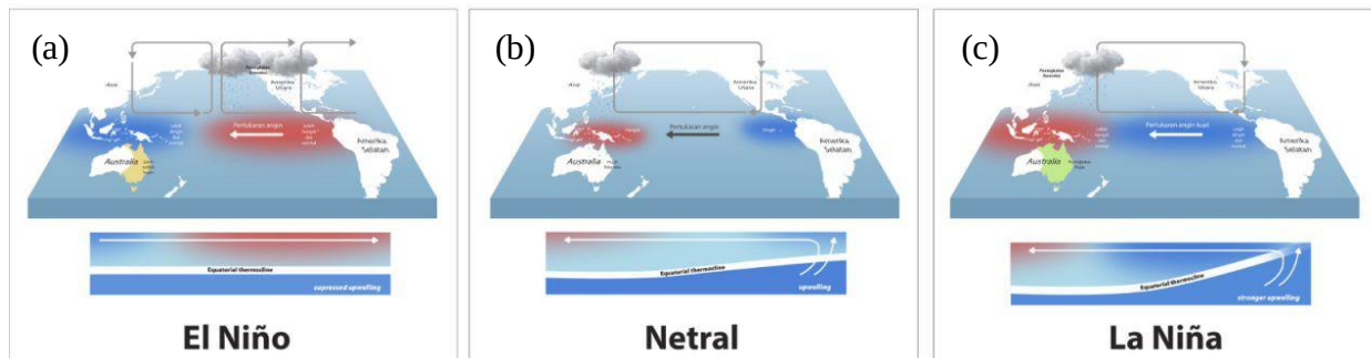
Gambar 1. (a) El Nino, (b) ENSO-netral, dan (c) La Nina (Sumber: www.bmkg.go.id )
