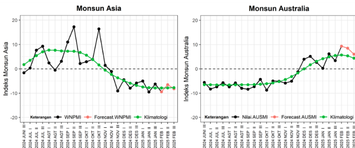
Gambar 8. Indeks Monsun Asia dan Indeks Monsun Australia di Wilayah Indonesia
