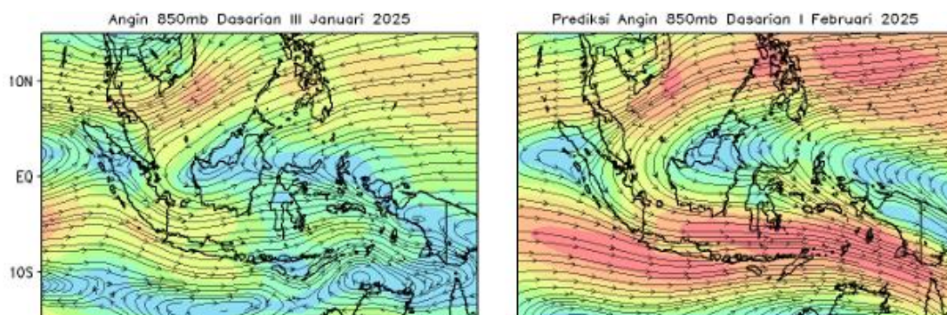
Gambar 7. Angin lapisan 850 mb di Wilayah Indonesia Dasarian III Januari 2025 dan Prediksi Angin 850 mb di Wilayah Indonesia Dasarian I Februari 2025 (Sumber : www.bmkg.go.id )
