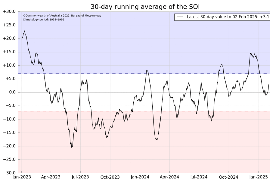
Gambar 6. Indeks SOI – 30 Harian (Sumber : www.bom.gov.au )
