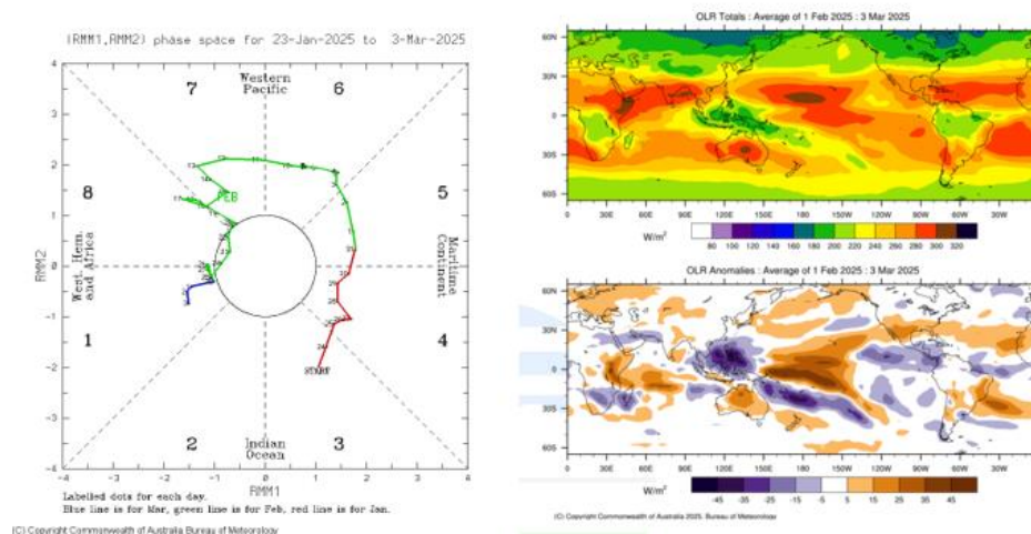
Gambar 9. Pergerakan MJO 23 Januari 2025 – 3 Maret 2025 (kiri) dan Total Rata-rata dan Anomali OLR 01 Februari 2025 – 03 Maret 2025 (kanan) (sumber: www.bom.gov.au )
