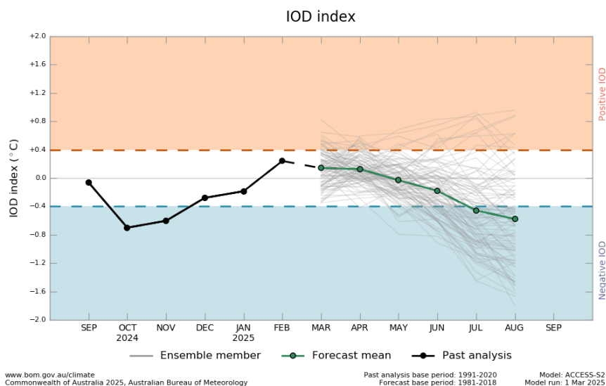
Gambar 5. Prediksi Indeks DMI
