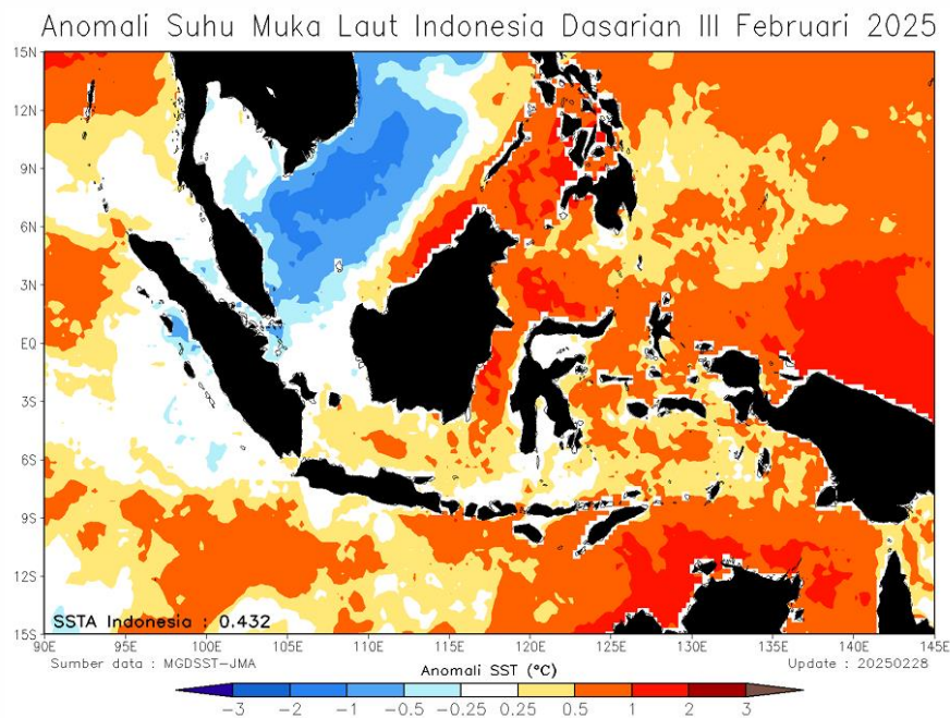
Gambar 11. Anomali SST Dasarian III Februari 2025 (sumber: www.bmkg.go.id )
