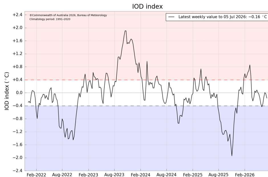
Gambar 4. Indeks DMI
