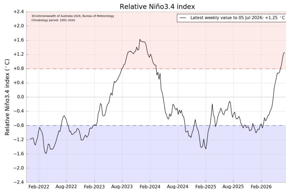
Gambar 2. Indeks Nino 3.4
