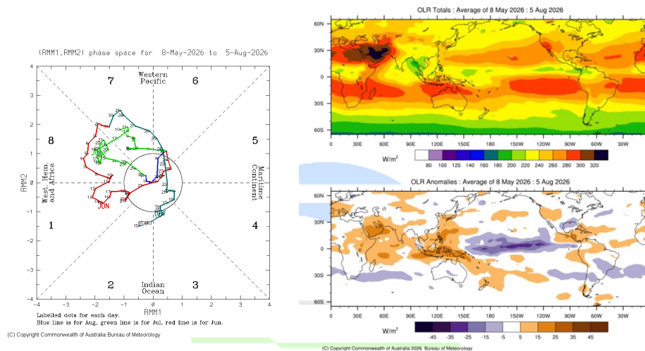
Gambar 9. Pergerakan MJO 8 Mei – 5 Agustus 2026 (kiri) dan Total Rata-rata dan Anomali OLR 8 Mei –5 Agustus 2026 (kanan) (sumber: www.bom.gov.au )
