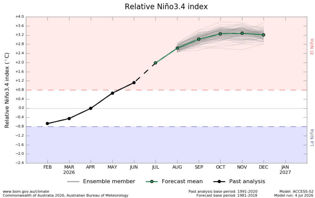
Gambar 3. Model Prediksi ENSO
