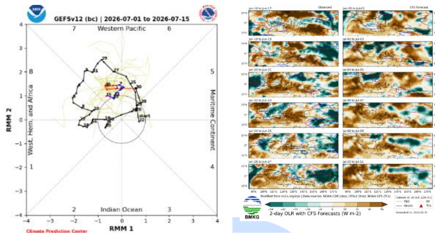
Gambar 10. Prediksi posisi MJO dan anomali OLR dasarian III Juni – II Juli 2026 (sumber: www.bmkg.go.id )
