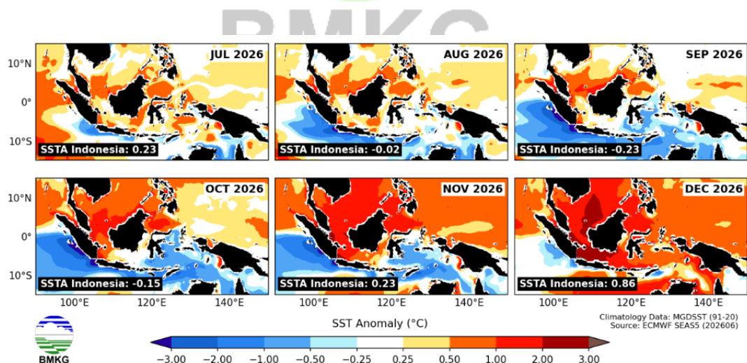
Gambar 12. Prediksi Anomali Juli 2026 – Desember 2026 (sumber: www.bmkg.go.id )
