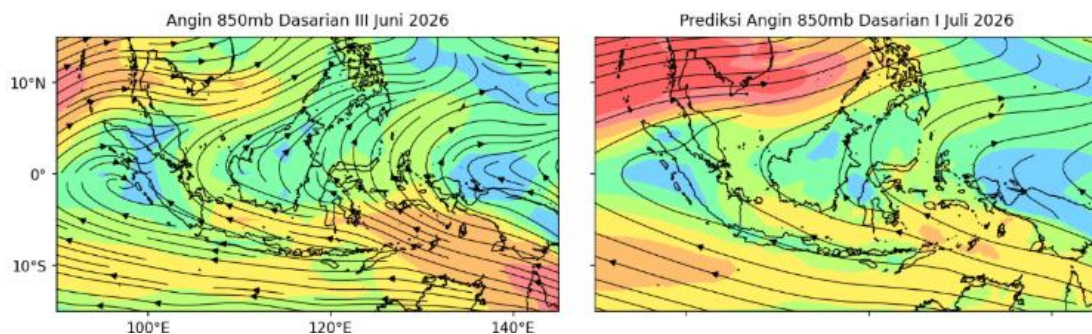
Gambar 7. Angin lapisan 850 mb di Wilayah Indonesia Dasarian III Juni 2026 dan Prediksi Angin 850 mb di Wilayah Indonesia Dasarian I Juli 2026
