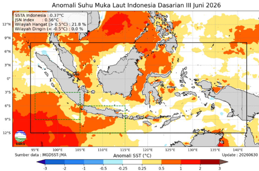
Gambar 11. Anomali SST Dasarian III Juni 2026 (sumber: www.bmkg.go.id )
