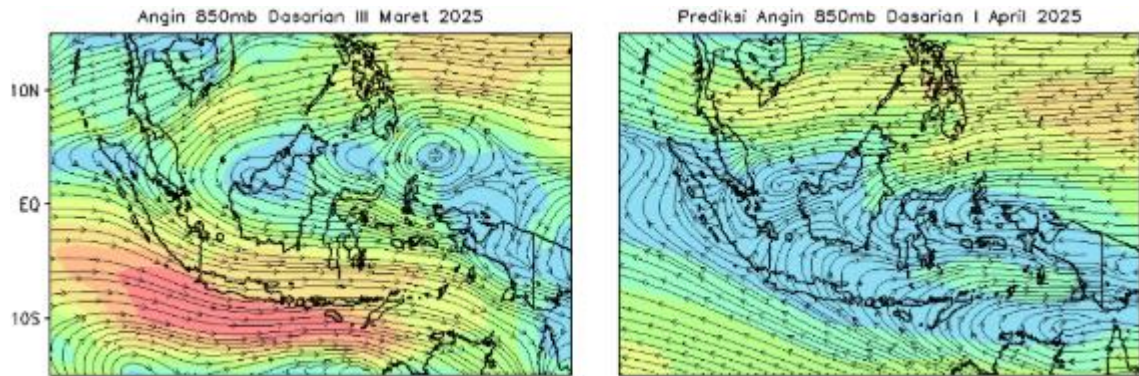
Gambar 7 : Angin lapisan 850 mb di Wilayah Indonesia Dasarian III Maret 2025 dan Prediksi Angin 850 mb di Wilayah Indonesia Dasarian I April 2025
