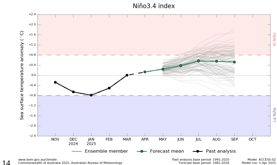
Gambar 3. Model Prediksi ENSO
