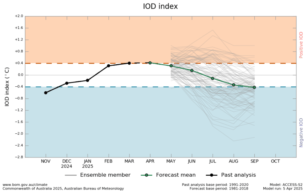
Gambar 5. Prediksi Indeks DMI
