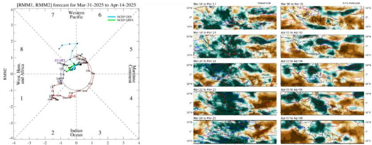
Gambar 9. Prediksi posisi MJO dan anomali OLR dasarian II Maret – II April 2025 (sumber: www.bmkg.go.id )
