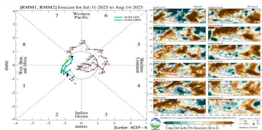
Gambar 10. Prediksi posisi MJO dan anomali OLR dasarian III Juli 2025 – II Agustus 2025 (sumber: www.bmkg.go.id )
