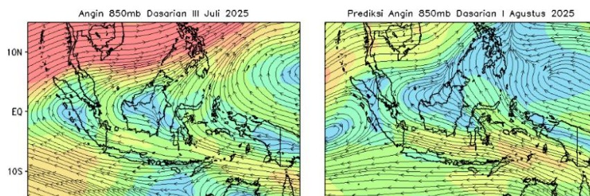
Gambar 7. Angin lapisan 850 mb di Wilayah Indonesia Dasarian III Juli 2025 dan Prediksi Angin 850 mb di Wilayah Indonesia Dasarian I Agustus 2025 (Sumber : www.bmkg.go.id )
