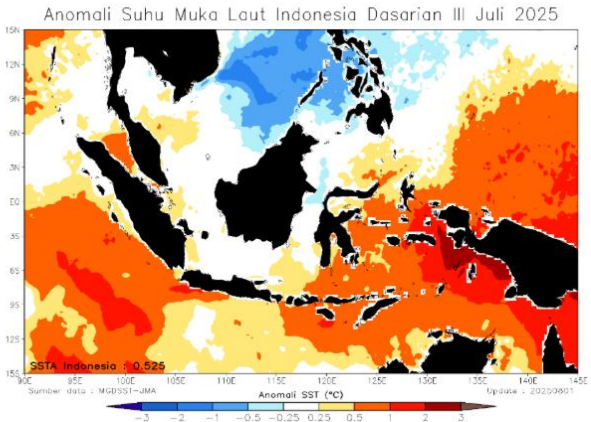
Gambar 11. Anomali SST Dasarian III Juli 2025 (sumber: www.bmkg.go.id )
