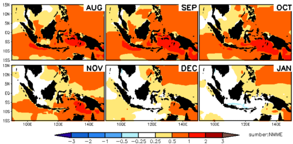
Gambar 12. Prediksi Anomali Agustus 2025 – Januari 2026 (sumber: www.bmkg.go.id )
