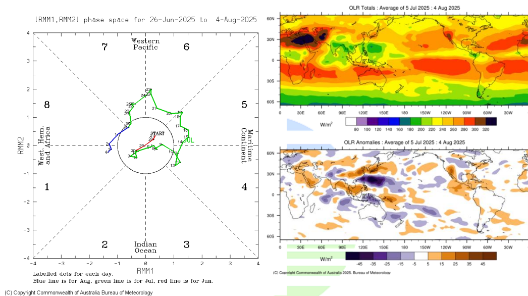
Gambar 9. Pergerakan MJO 26 Juni 2025 – 4 Agustus 2025 (kiri) dan Total Rata-rata dan Anomali OLR
