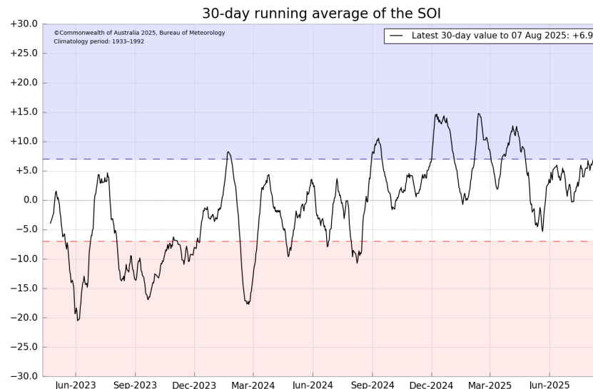
Gambar 6. Indeks SOI – 30 Harian (Sumber : www.bom.gov.au )
